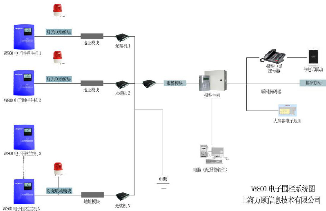
脉冲电子围栏专用控制主机组网系统图
