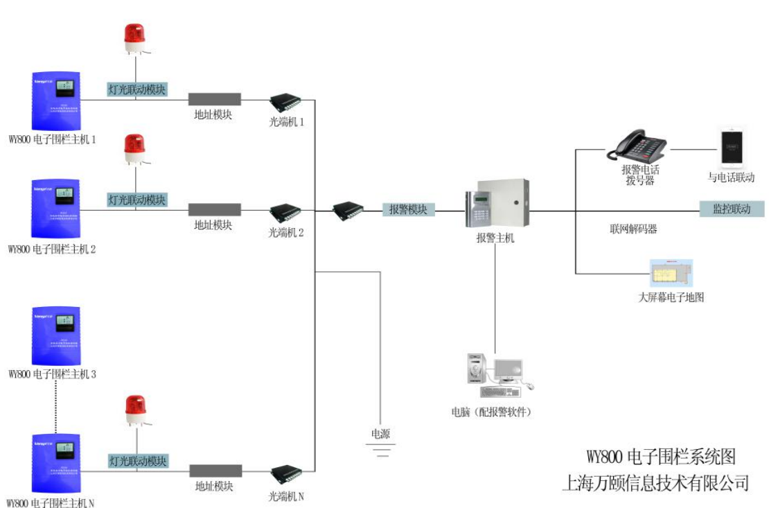
典型电子围栏组网系统图
